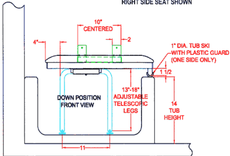
CA416-2SD (R / L)
